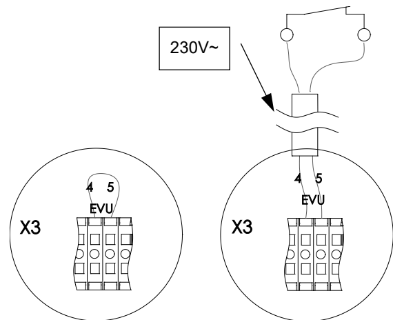
Abbildung 5: EVU Meldekontakt
