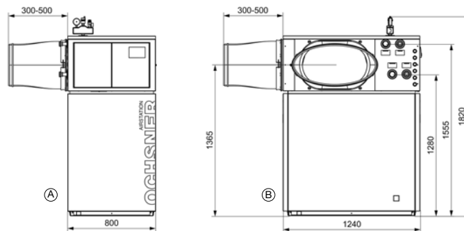
(A) Vorderansicht (B) Seitenansicht
